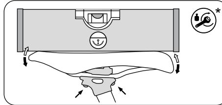
Patentstütze mit Zweischraubenbefestigung
