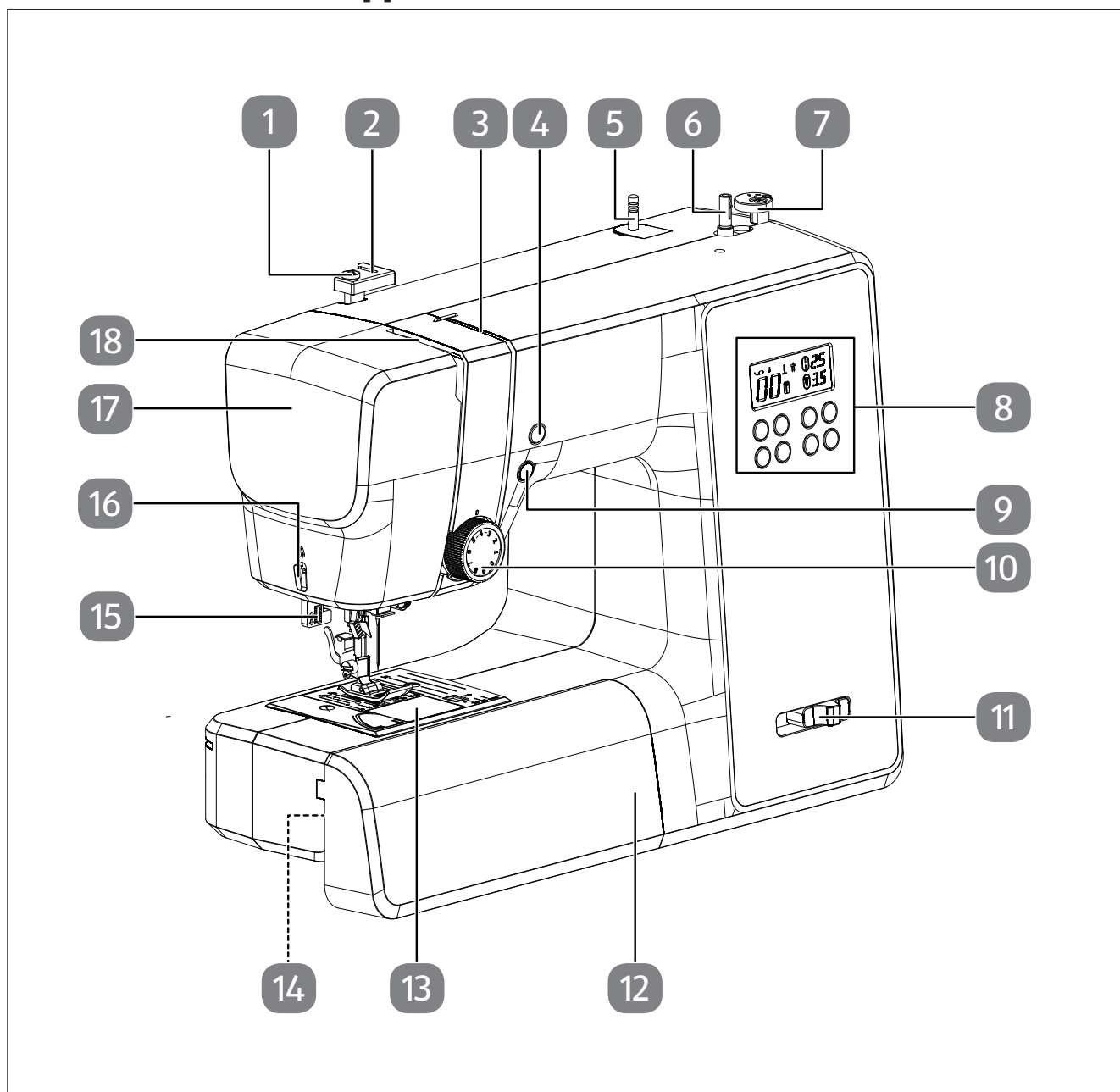
Afb. 1 – Vooraanzicht
