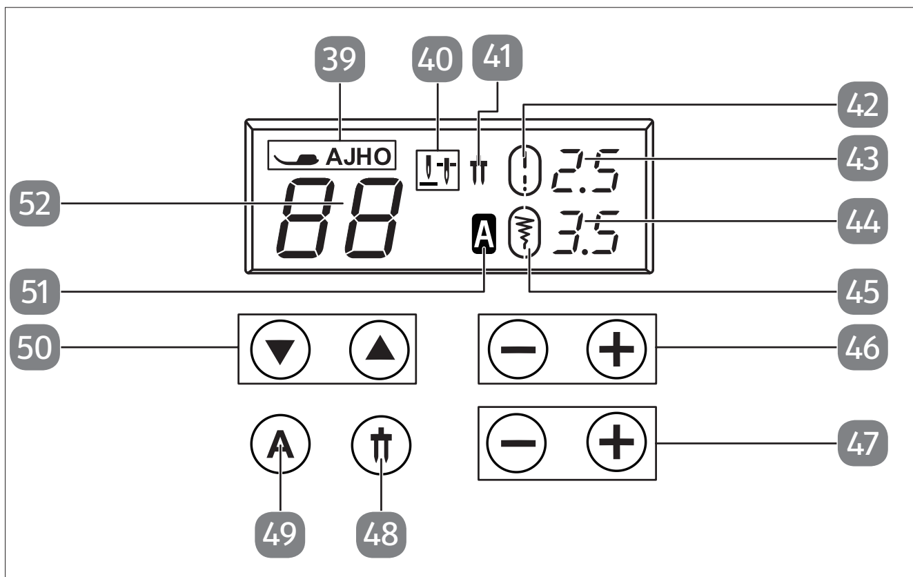
Abb. 4 – Display und Bedienfeld
