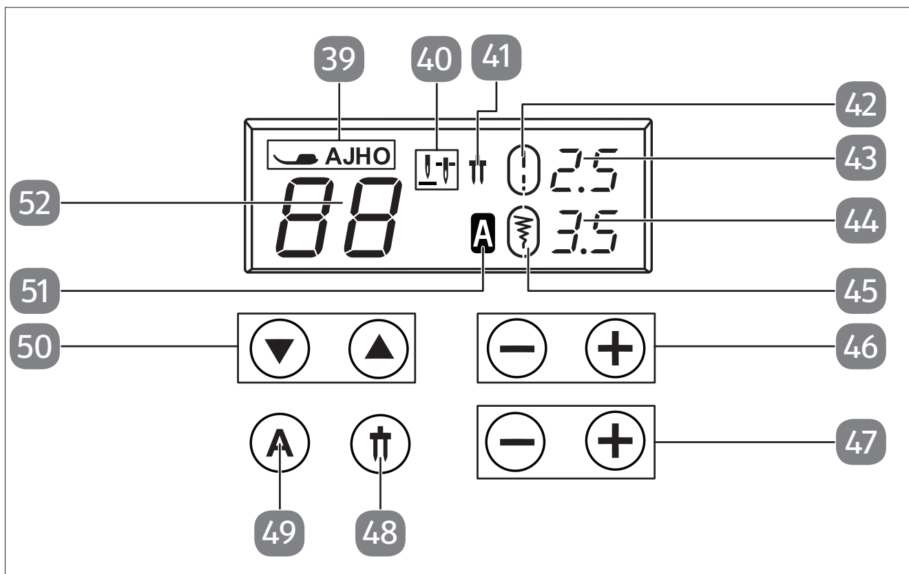
Fig. 4 – Pantalla y panel de control
