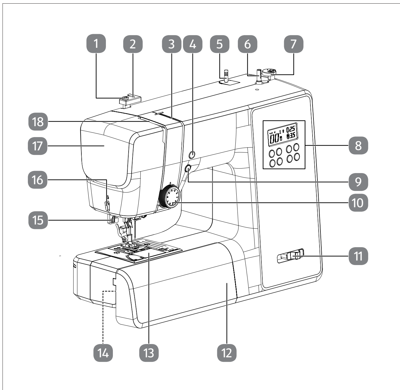
Abb. 1 – Vorderansicht
